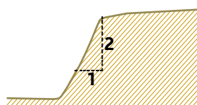
Pente de talutage 1/2
